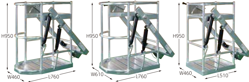
G-01 先丸小 アブソーバー式 G-02 先丸大 アブソーバー式 G-03 角小 アブソーバー式
