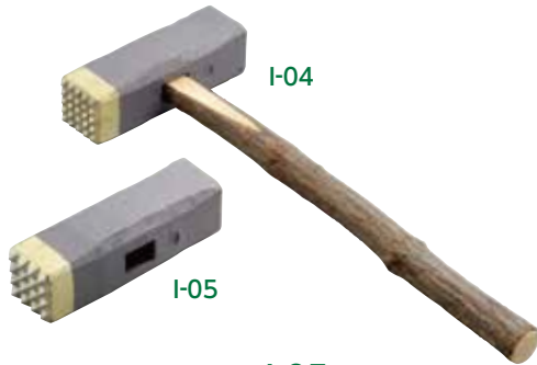
I-04 近藤 ビシャン片刃 5×5×25刃 (うしごろし柄付)
